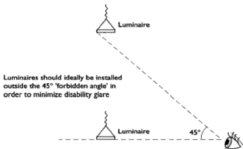
محل مطلوب نصب منابع روشنایی
